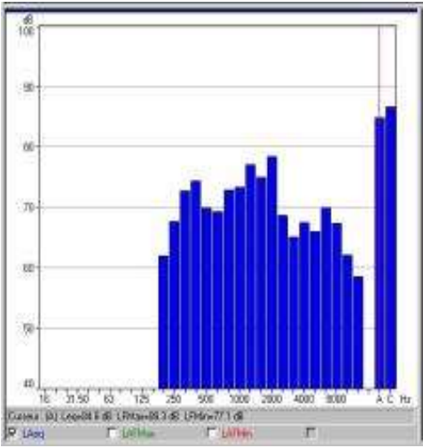
Fast punch press 85 dB(A)
